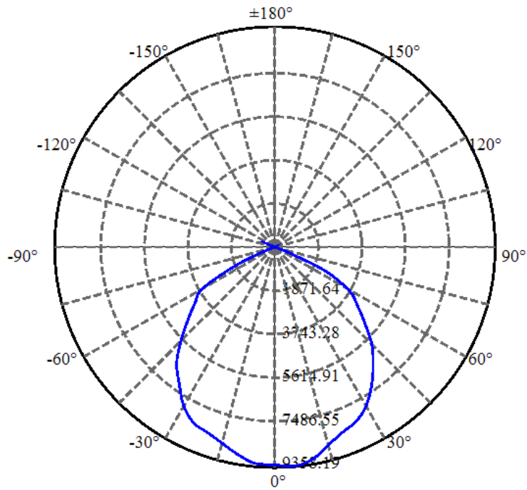
直角座標圖 C90 / 270
